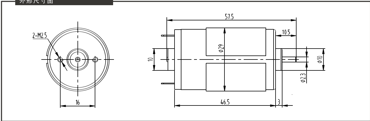
马达参数
